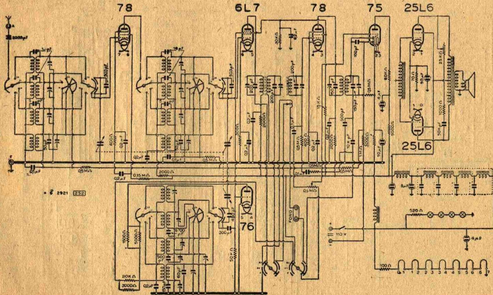
Lo schema elettrico del radiofonaografo mod. «748 cc» a corrente continua.
